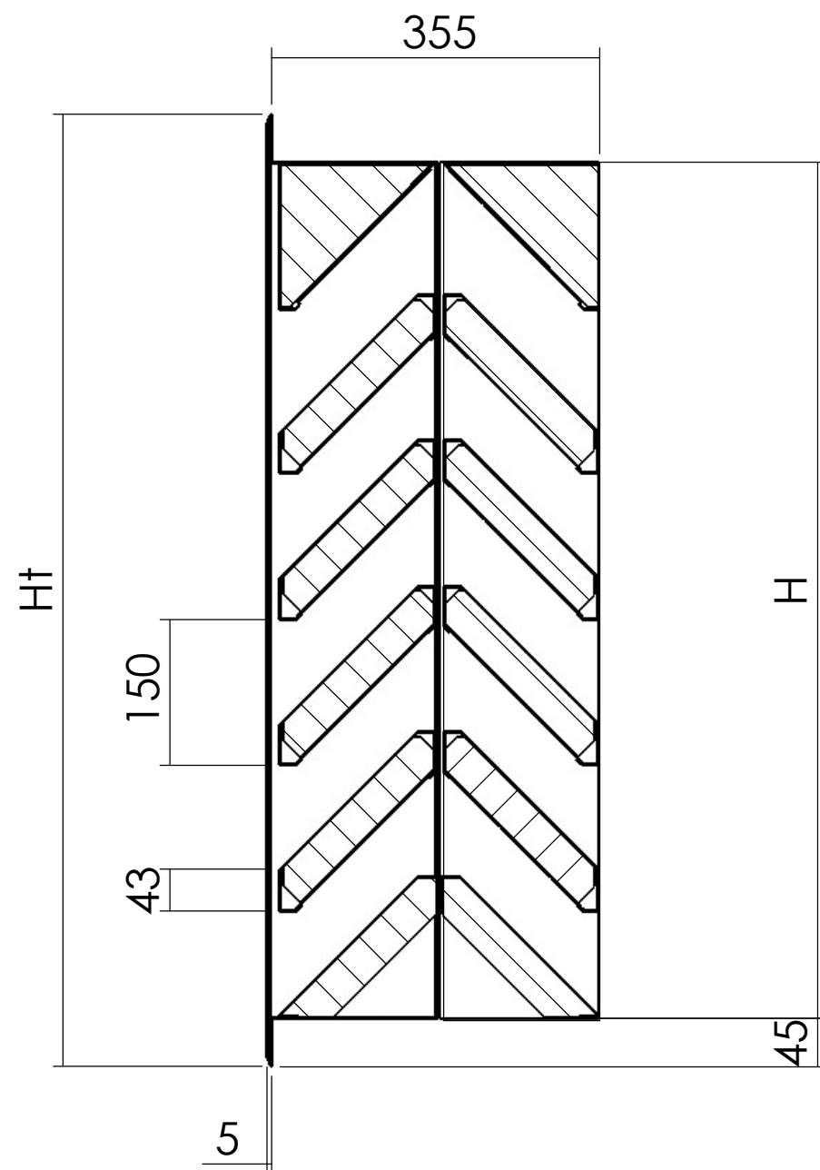
SECTION A-A
