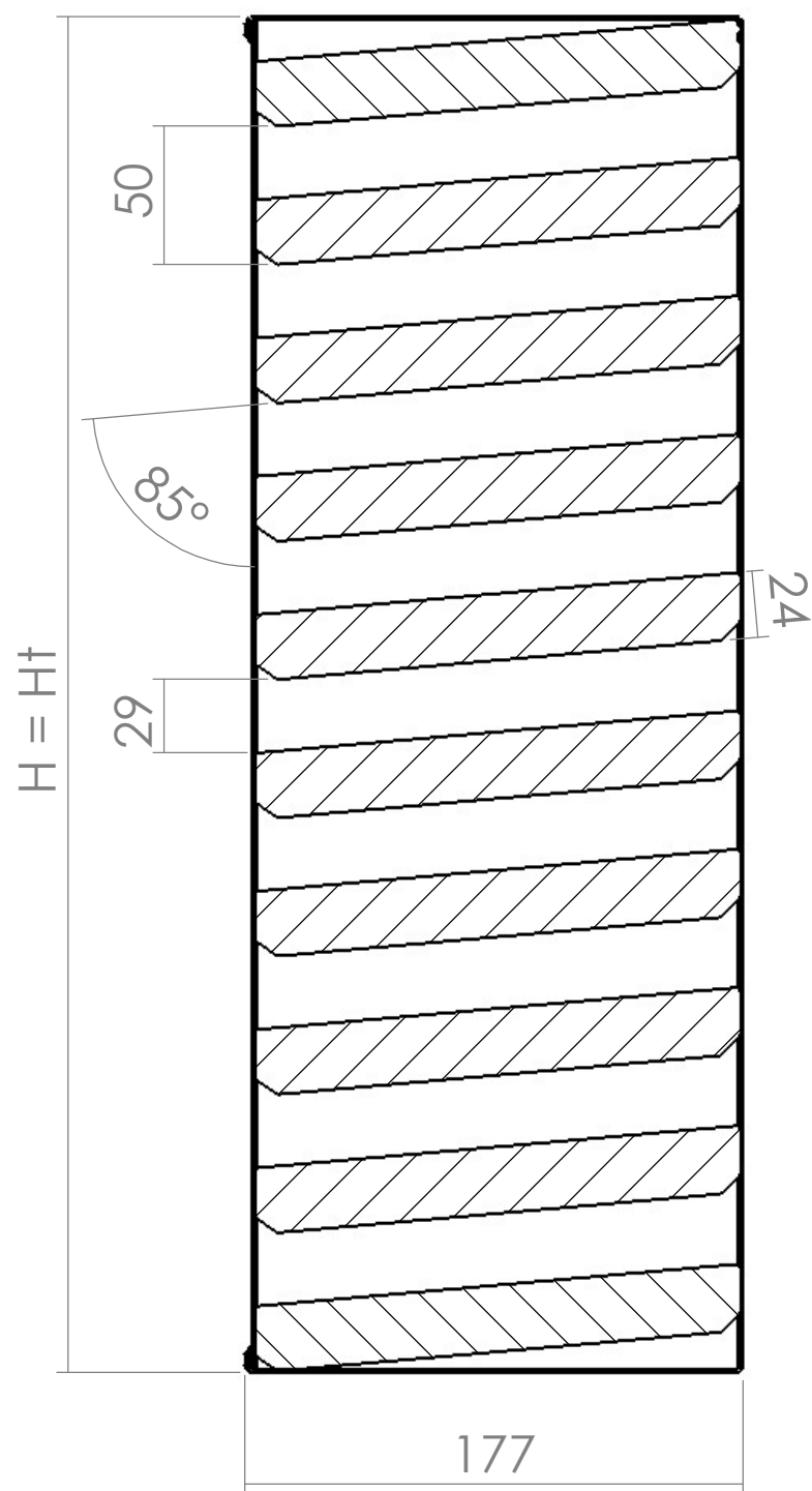
SECTION A-A SCALE 1 : 4
