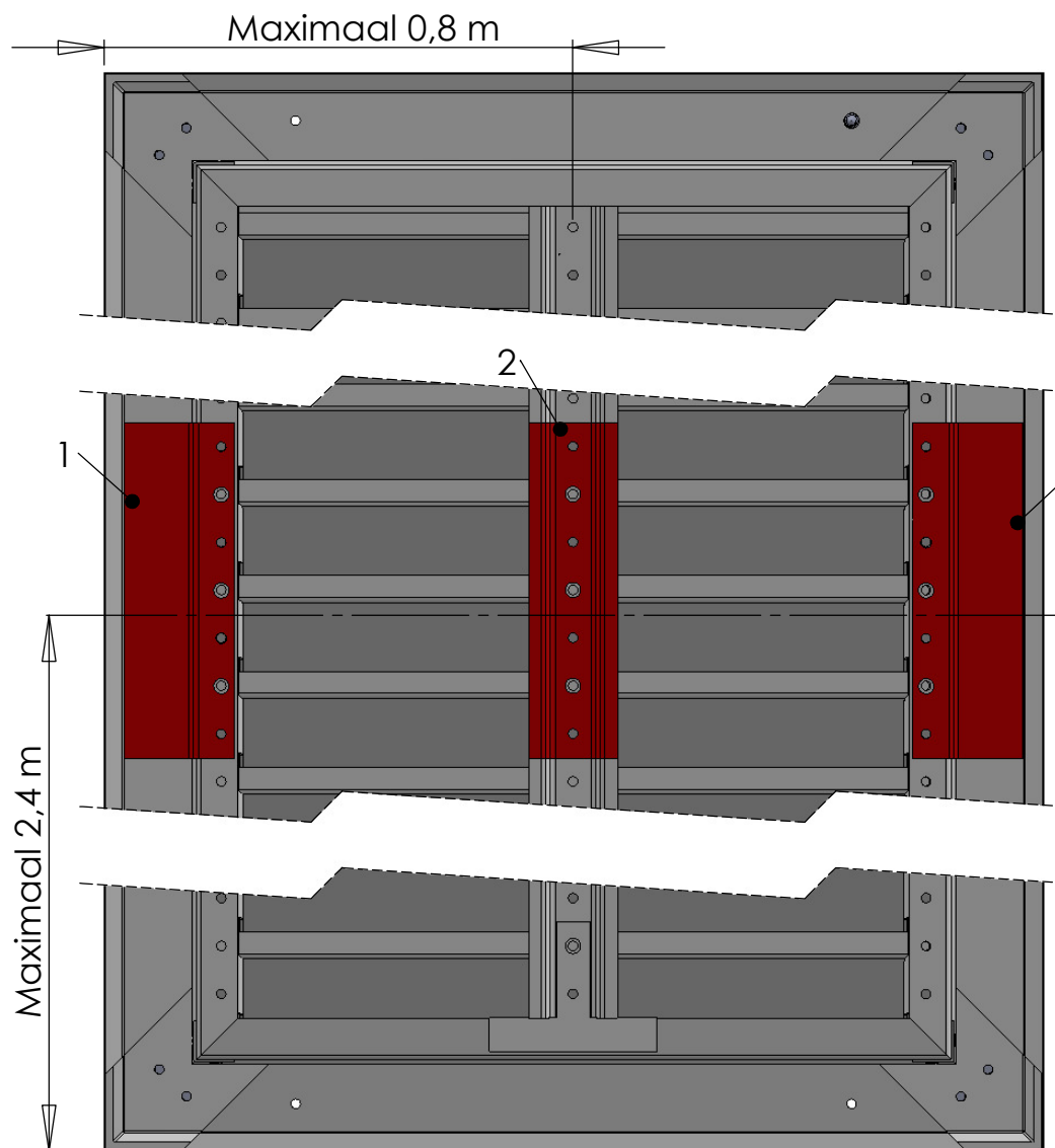
Achteraanzicht
