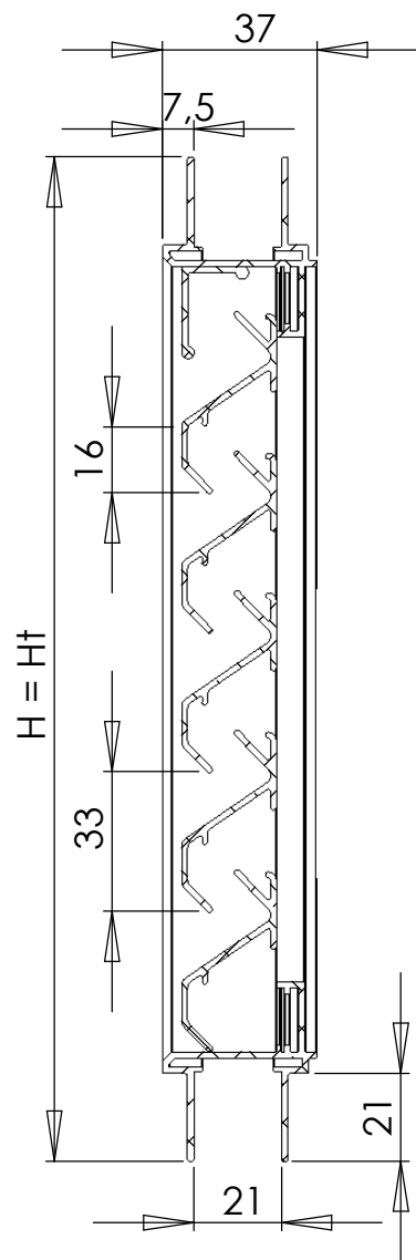
SECTION A-A SCALE 1 : 2
