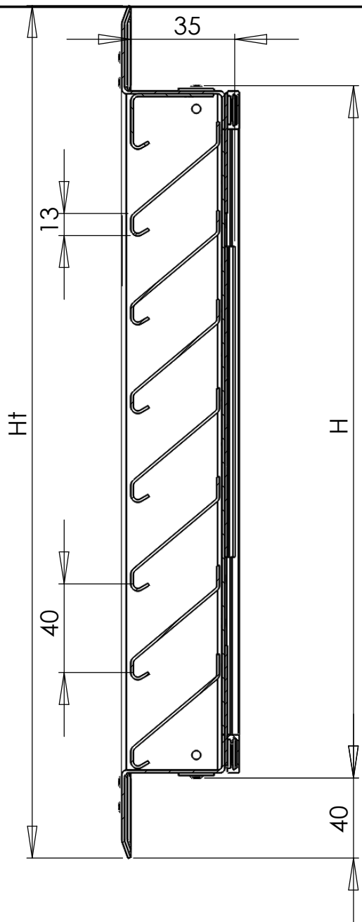
SECTION A-A
