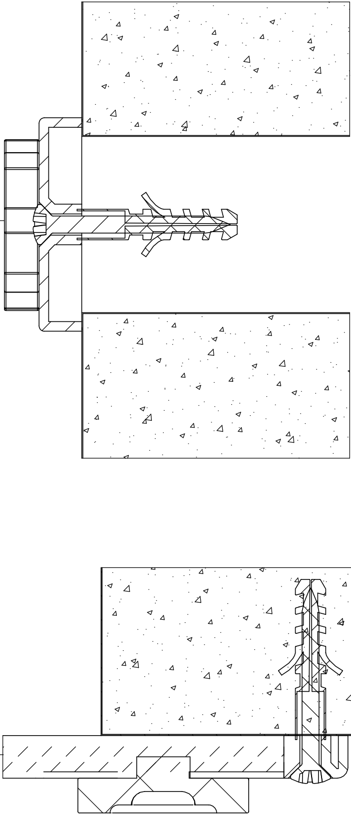
Fixation
